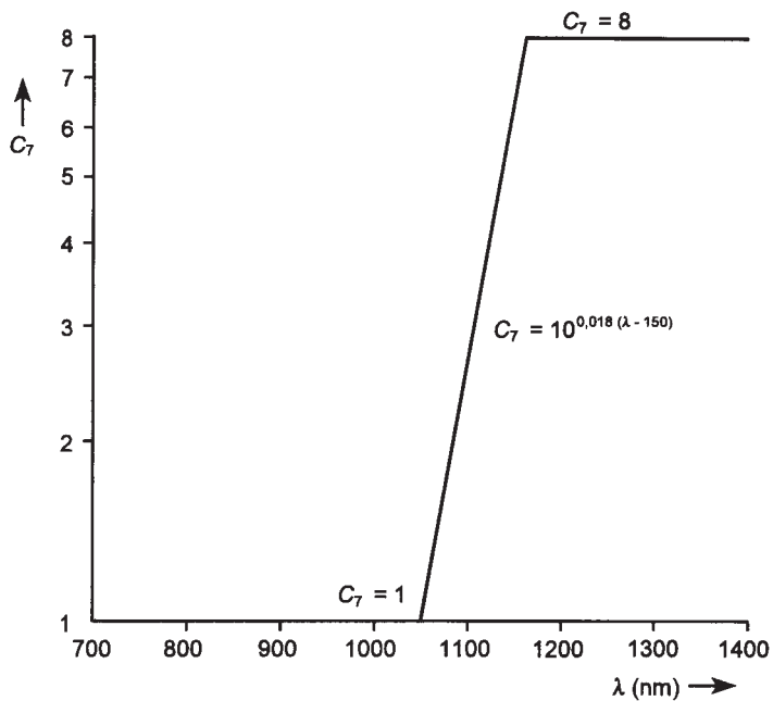
Bild 8: Korrekturfaktor C_7 für \lambda = 1050 nm bis 1400 nm
