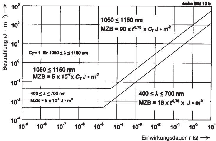
Bild 10a: MZB für direkte Bestrahlung des Auges ( C_6 = 1 ) durch sichtbare ( 400 \text{ nm} \leq \lambda < 700 \text{ nm} ) und ausgewählte Infrarot-Strahlung ( 1050 \text{ nm} \leq \lambda < 1150 \text{ nm} ), direkter Blick in den Strahl, für Einzelimpulse oder Bestrahlungen (Expositionen)
