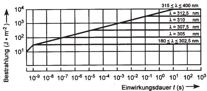
Bild 9b: MZB für direkte Bestrahlung des Auges durch UV-Strahlung für Einwirkungsdauern bei ausgewählten Wellenlängen
