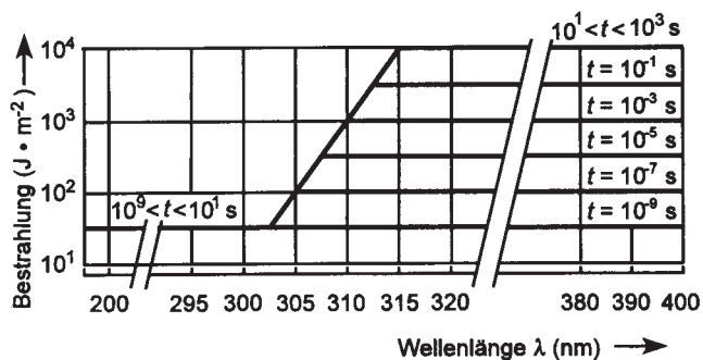
Bild 9a: MZB für direkte Bestrahlung des Auges durch UV-Strahlung bei ausgewählten Emissionsdauern von 10^{-9} bis 10^3 \text{ s}
